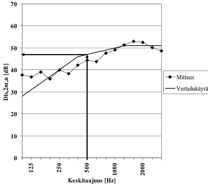
Kuva 2. Yksilukuisen normalisoidun äänitasoeroluvun määrittäminen vertailukäyrämenettelyllä kuvassa 1 esitetyistä mitatuista normalisoiduista äänitasoeroista. Normalisoitu äänitasoeroluku on 47 dB.
