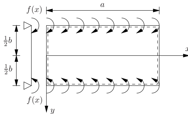
Kuva 9.5 Vapaasti tuetun laatan akselin x suhteen symmetrinen reunamomentti-kuorma.
