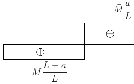
Kuva 2.5 Vääntömomenttikuvio.
