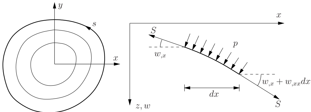
Kuva 2.25 Kalvon taipuma.
