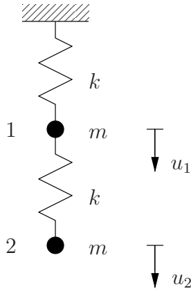
Kuva 1.12 Kahden jousen ja massan systeemi.
