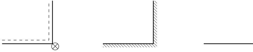
Kuva 7.9 a) Vapaasti tuettu, b) kiinnitetty ja c) vapaa laatan nurkka.
