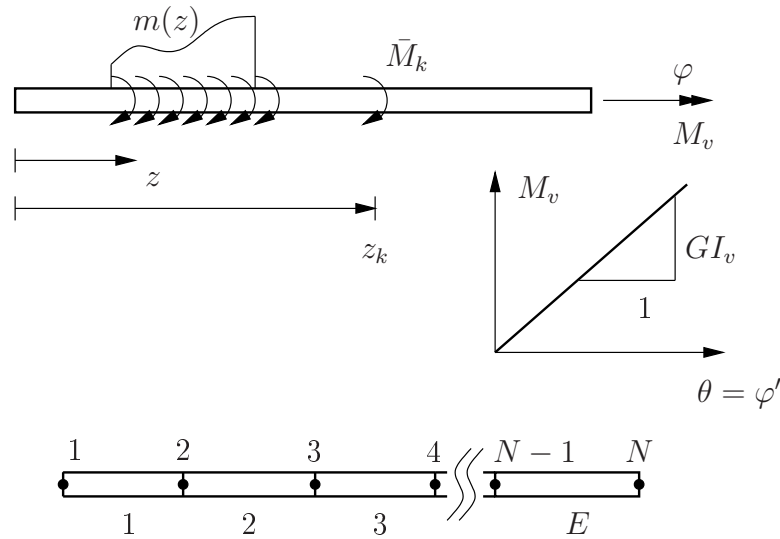
Kuva 2.6 Vääntösauvan elementtimalli.
