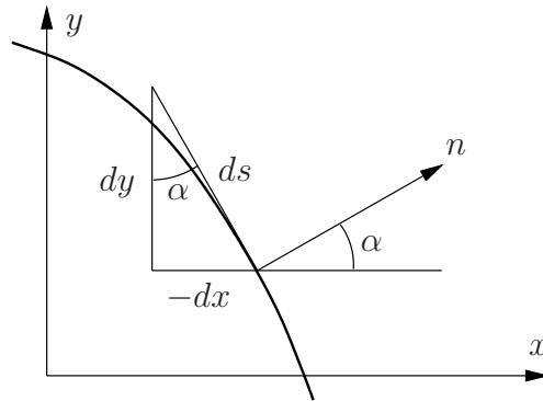
Kuva 4.2 Poikkileikkauksen seinämän tangentti ja normaali.
