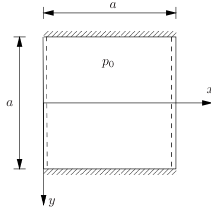
Kuva 9.8 Akselin x suuntaisilta reunoilta kiinnitetty neliölaatta.
