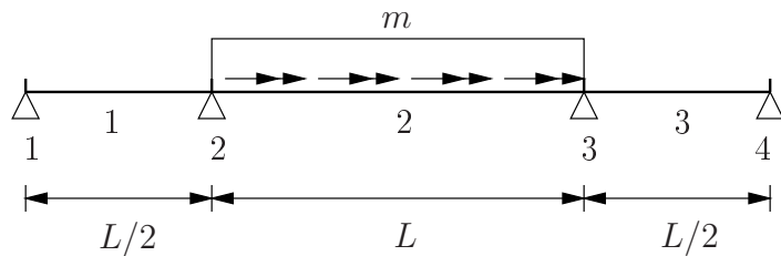
Kuva 5.5 Symmetrinen kolmiaukkoinen vääntösauna.
