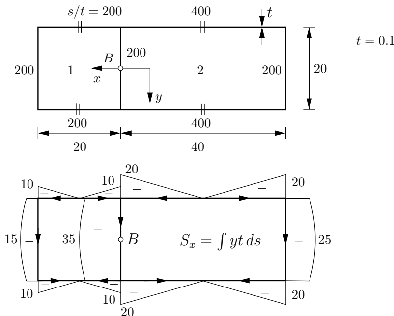
Kuva 6.2 Kaksikoteloinen poikkileikkaus.
