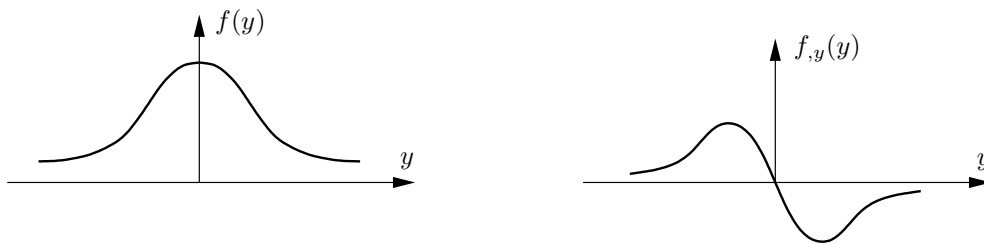
Kuva 10.6 Symmetrinen funktio.
