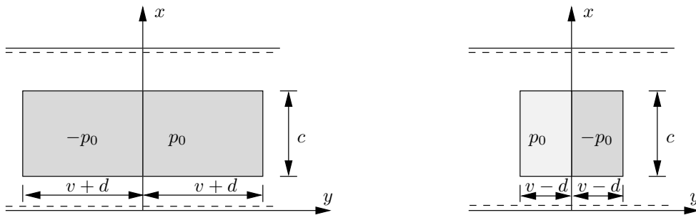
Kuva 10.12 Antisymmetriset palakuormat.
