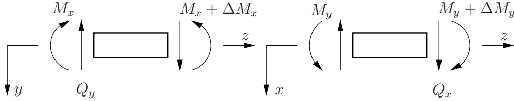
Kuva 4.17 Taivutusmomenttien M_x ja M_y merkkisäännöt.
