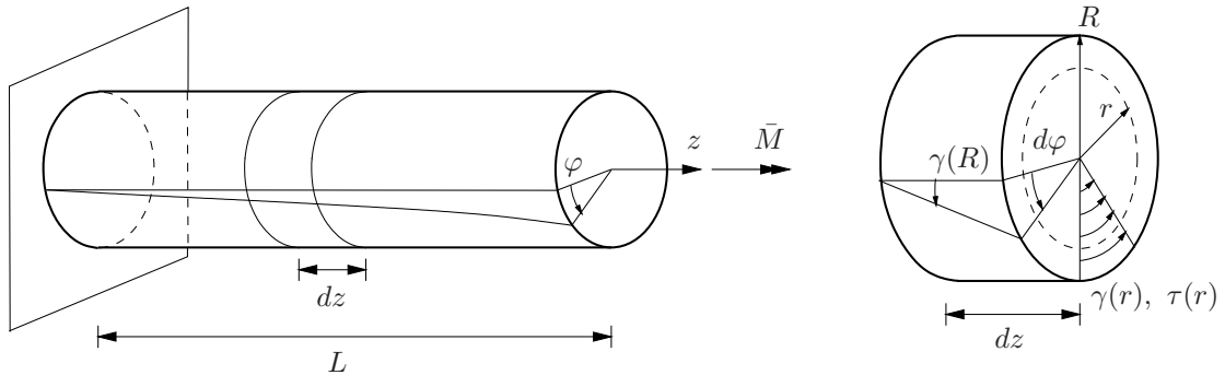
Kuva 2.1 Pyöreän ulokesauvan vääntö.
