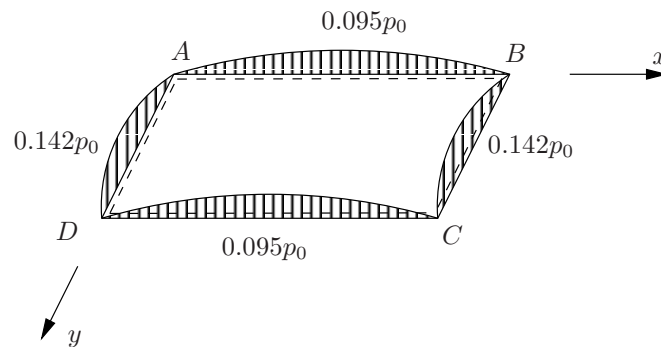
Kuva 8.7 Vääntömomentin derivaatta M_{ns,s} .
