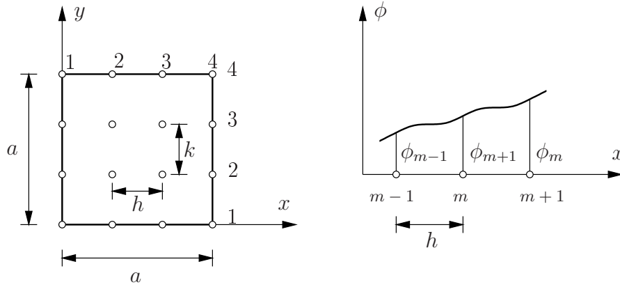
Kuva 2.18 Differenssimenetelmän hila.
