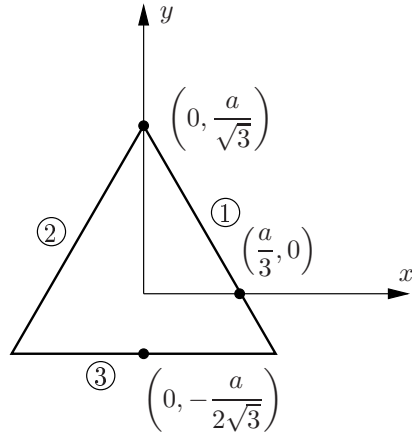
Kuva 2.14 Tasasivuisen kuolmion muotoinen poikkileikkaus.
