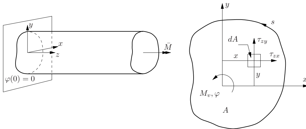
Kuva 2.21 Ulokesauvan vääntö.
