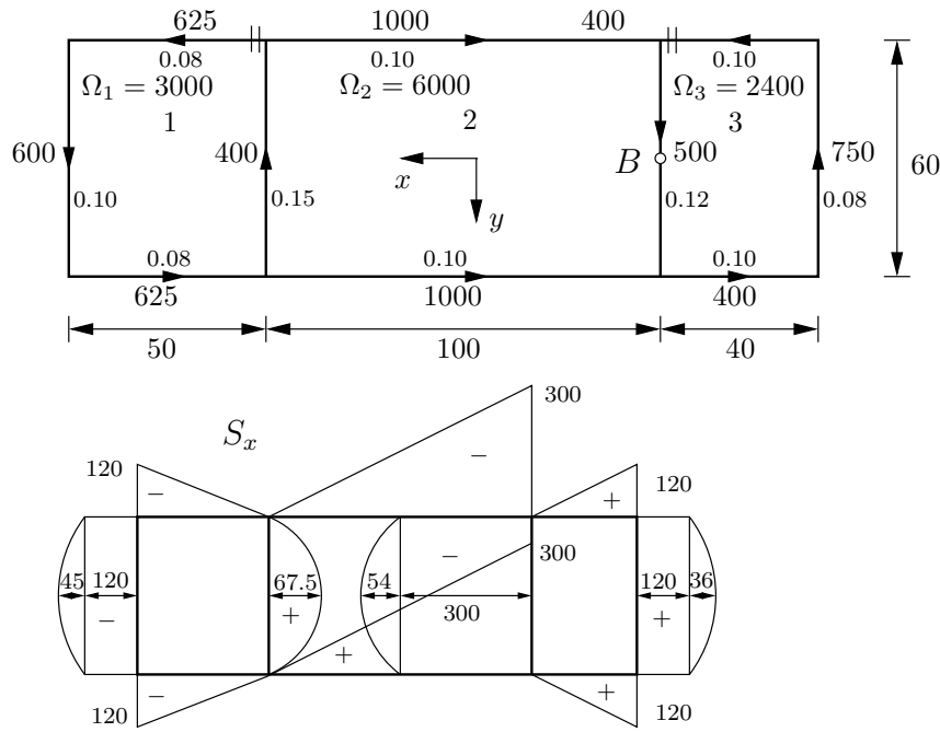
Kuva 6.4 Kolmikoteloinen poikkileikkaus.
