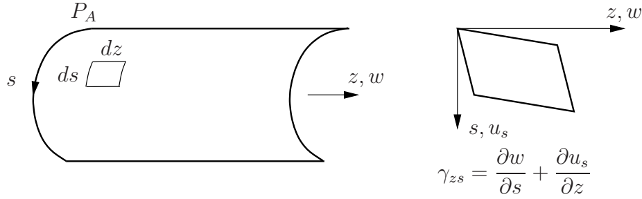
Kuva 4.3 Seinämän keskipinnan koordinaatisto (s, z) ja liukuma \gamma_{sz} .
