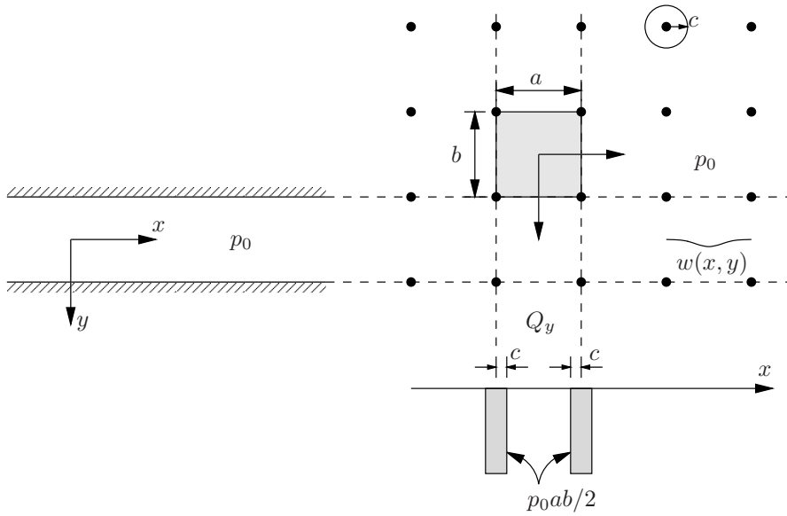
Kuva 9.11 Pilarilaatta.
