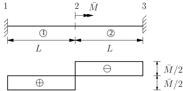
Kuva 2.10 Elementtimenetelmällä ratkaistu vääntömomenttikuvio.
