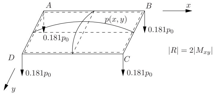
Kuva 8.5 Nurkkavoimat.
