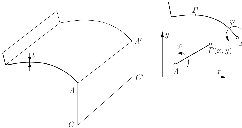
Kuva 5.11 Tasossaan jäykän levyn tukema katos, jonka reunat ovat nivelelliset.
