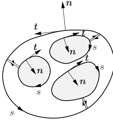
Kuva 2.13 Onteloita sisältävä poikkileikkaus.
